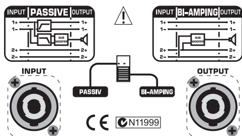
Рис. 1.1: Панель подключений сабвуфера (E1800X)
