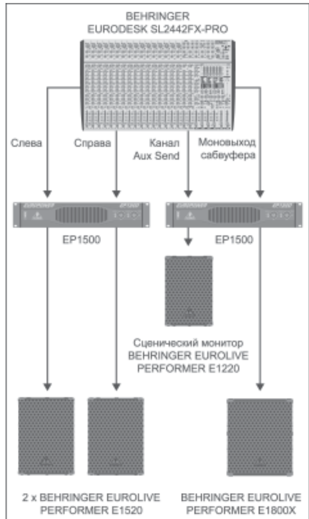
Рис. 6.1: Стереорежим со сценическим монитором и сабвуфером
