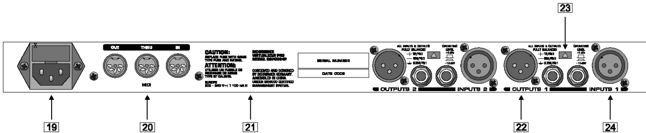
Рис. 1.4: Задняя панель VIRTUALIZER PRO
